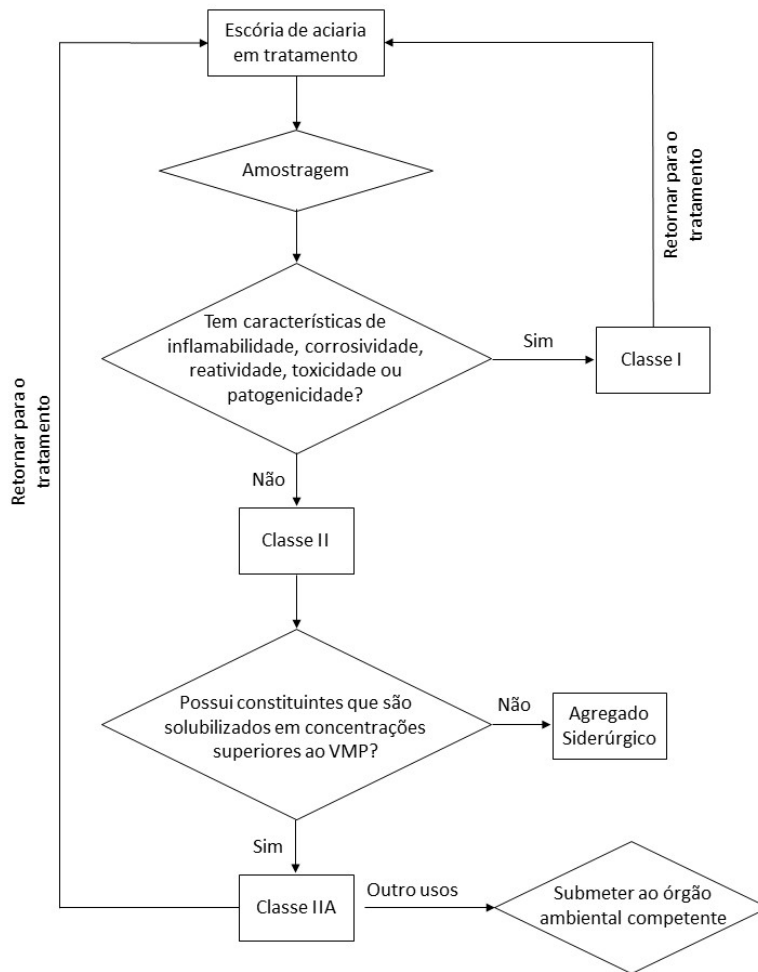
Fluxograma de caracterização e classificação do Agregado Siderúrgico (Adaptado da Norma ABNT NBR 10004/2004)
