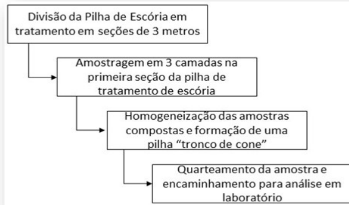
Figura 3 – Esquema geral do processo de amostragem
